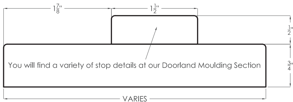
FLAT JAMB
