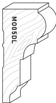
MO05DL 1\text{-}\frac{3}{4}'' \times 3\text{-}\frac{3}{4}'' 44mm x 95mm
